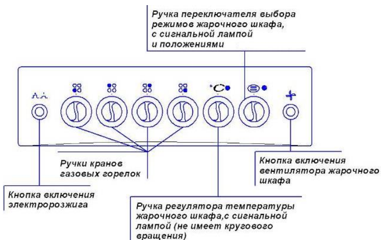
Рис. 11 Передняя панель плиты с электрическим жарочным шкафом
