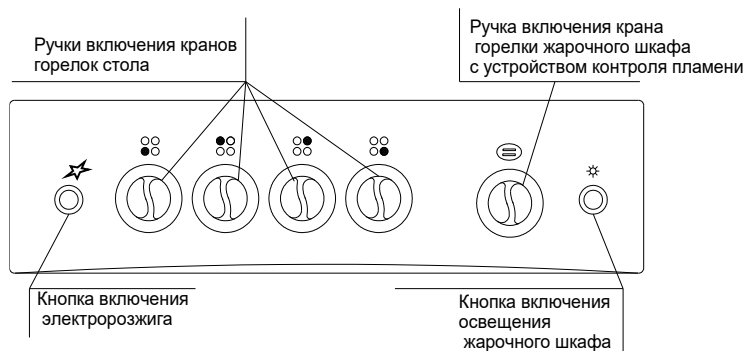
Рис. 10 Передняя панель плиты с газовым духовым шкафом
