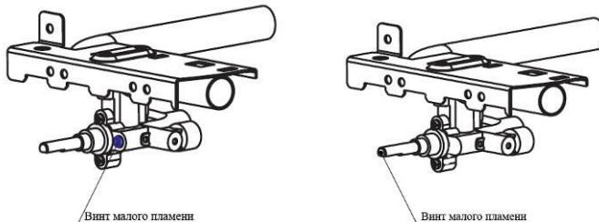
Рис. 8. Возможное расположение винтов малого пламени.
